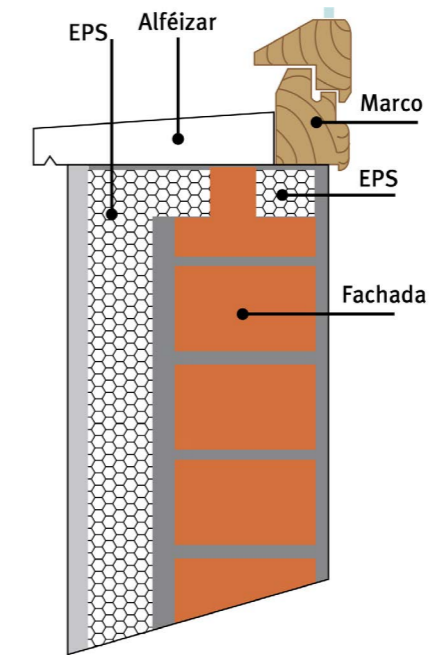
Fig. 19. Detalle 2. Sistema SATE. Encuentro de fachada con alféizar.
