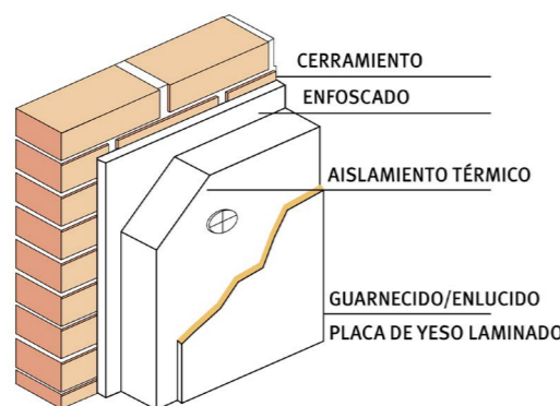
Fig. 9. Esquema del trasdosado con placa de yeso laminado
