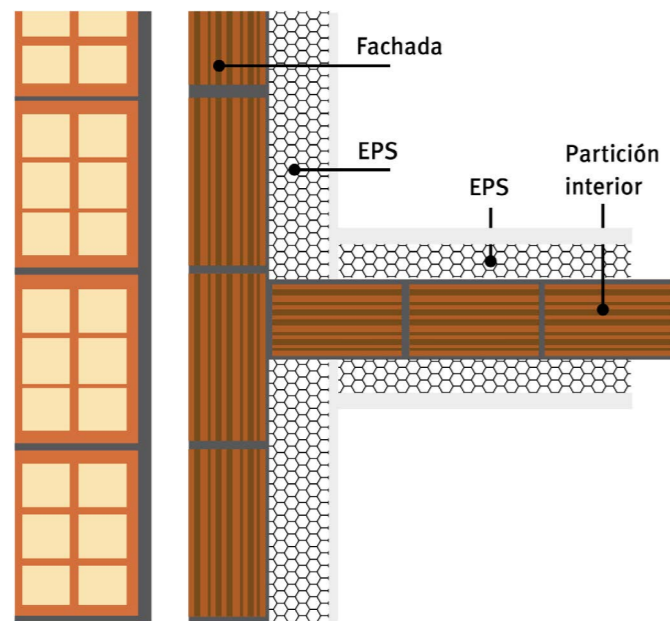
Fig. 29. Detalle 4. Aislamiento térmico por el interior. Encuentro de fachada con particiones interiores.
